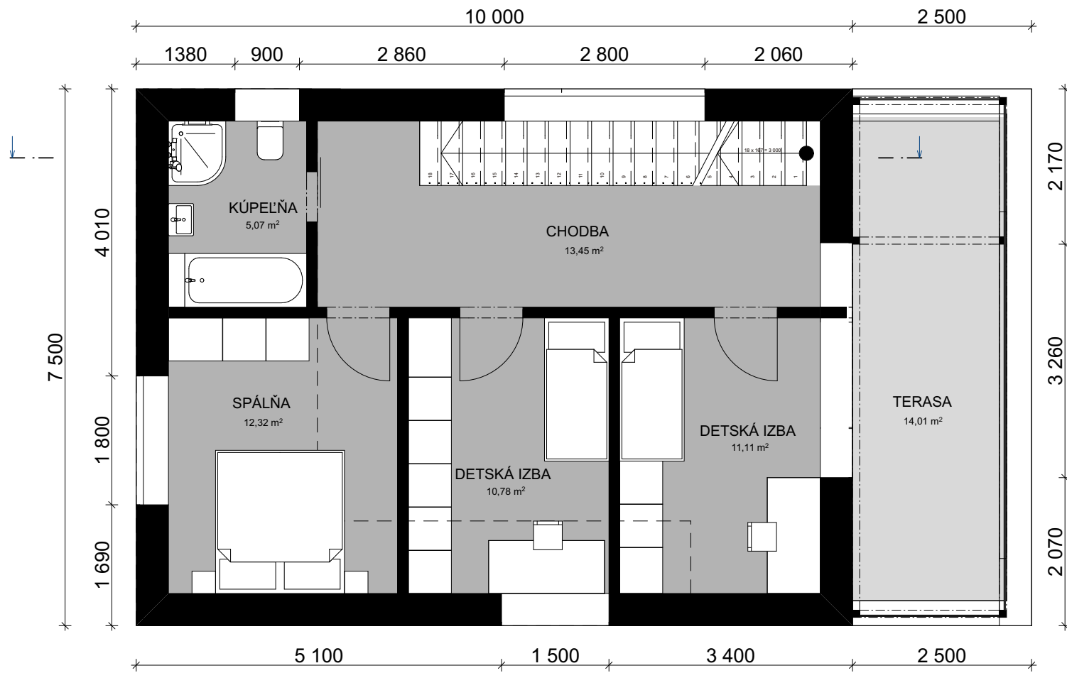
pôdorys 2np
